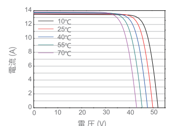
電流-I-Vカーブ JAM72D30-540/MB
