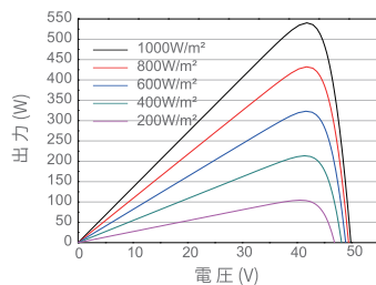
出力-I-Vカーブ JAM72D30-540/MB
