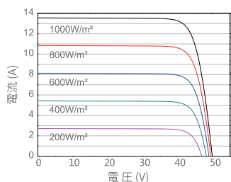
電流-I-Vカーブ JAM72D30-540/MB
